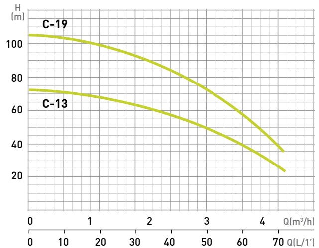
CS4 C-... JELLEGGÖRBÉK
