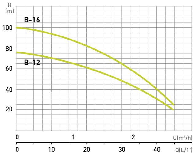
CS4 B-... JELLEGGÖRBÉK
