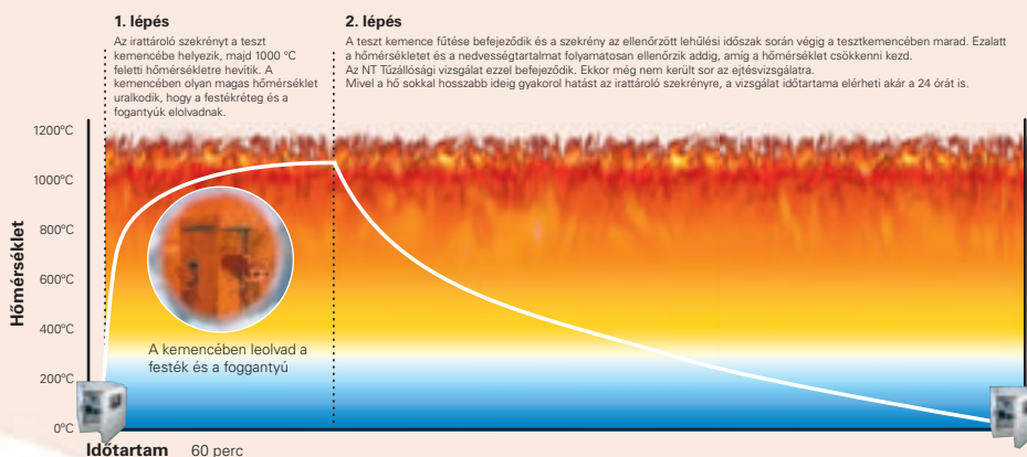
1. ábra: EN 1047, UL-72 szerint végzett vizsgálatok
