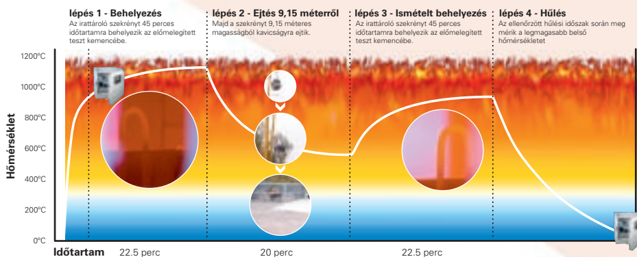
2. ábra: EN 1047-1, UL-72 vizsgálat
