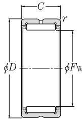
RNA49 · R type, RNA59 type RNA69 · R type ( \phi F_w \leq 35\text{mm} ) NK · R type
