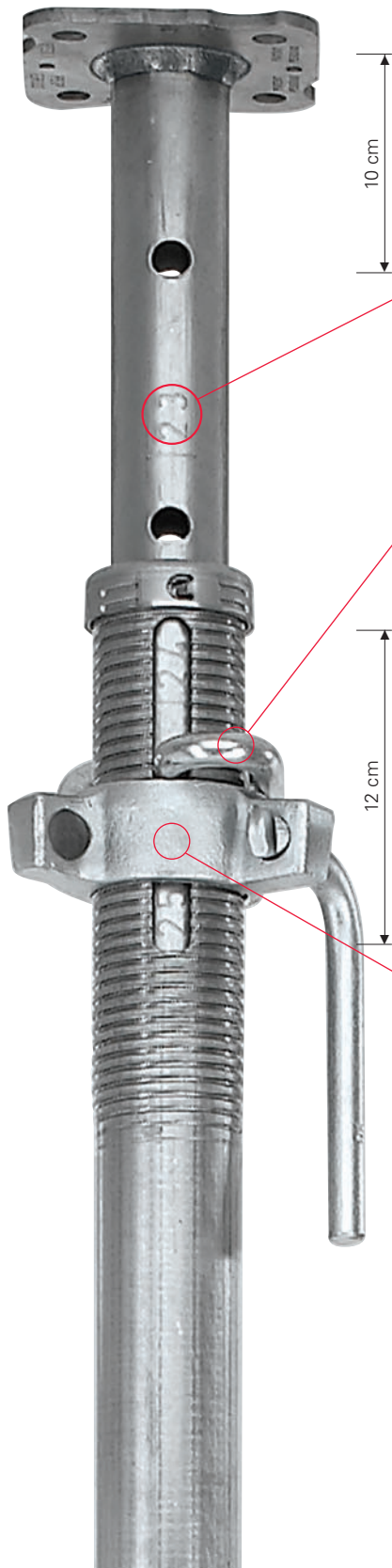
A méretjelölések könnyen olvashatóak a PEP Ergo támaszokon.
