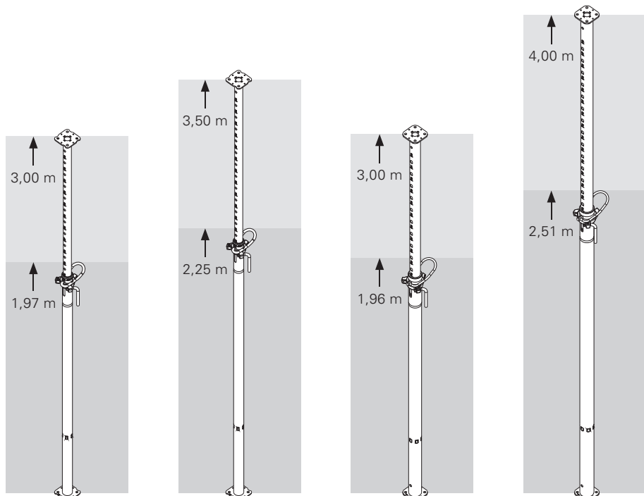
B-300 L = 1,97 – 3,00 m Súly: 14 kg B-350 L = 2,25 – 3,50 m Súly: 15,6 kg E-300 L = 1,96 – 3,00 m Súly: 19,4 kg E-400 L = 2,51 – 4,00 m Súly: 26,6 kg
