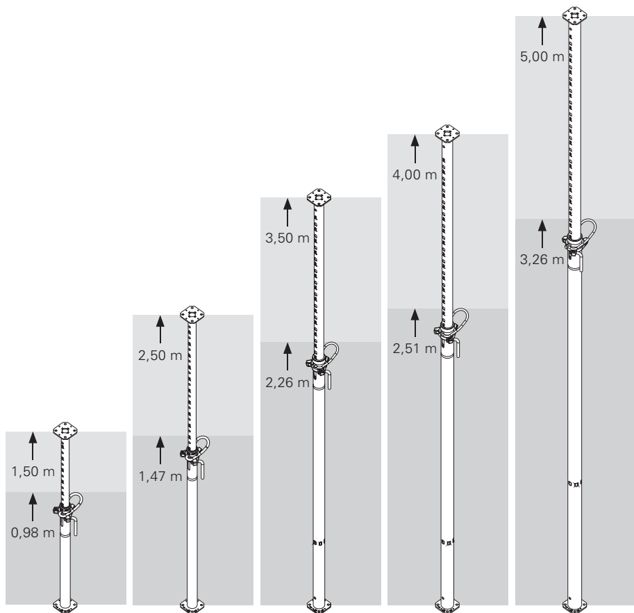
D-150 L = 0,98 – 1,50 m Súly: 9,1 kg D-250 L = 1,47 – 2,50 m Súly: 13,1 kg D-350 L = 2,26 – 3,50 m Súly: 19,7 kg D-400 L = 2,51 – 4,00 m Súly: 23,2 kg D-500 L = 3,26 – 5,00 m Súly: 30,7 kg
