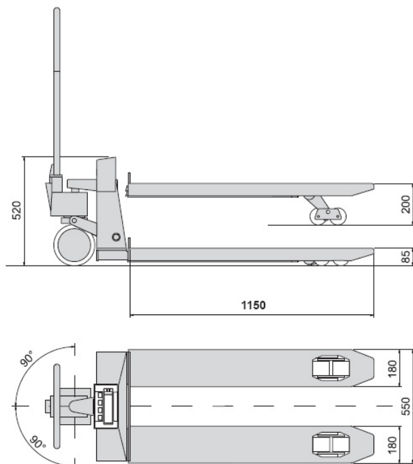
Méreték [mm]
