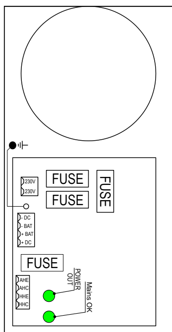
LINTAP2-12V/1A, LINTAP2-12V/2A Bekötési ábra
