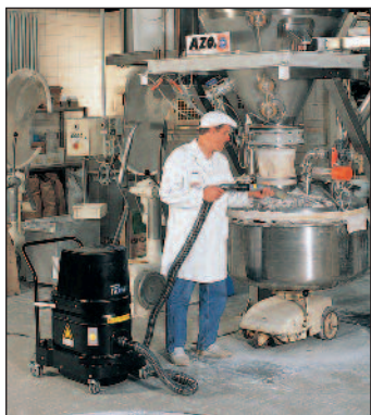
DS 1220 M 22 zóna
