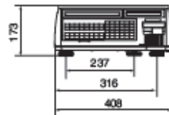
CL5000J-CB
