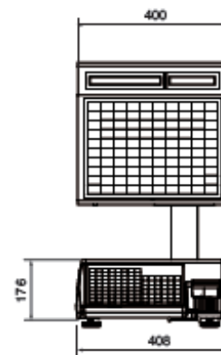
CL5000J-CS
