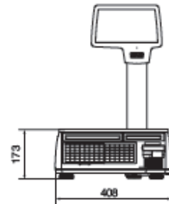
CL5000J-CR
