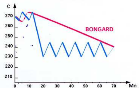
Összehasonlító hőmérsékleti görbék
